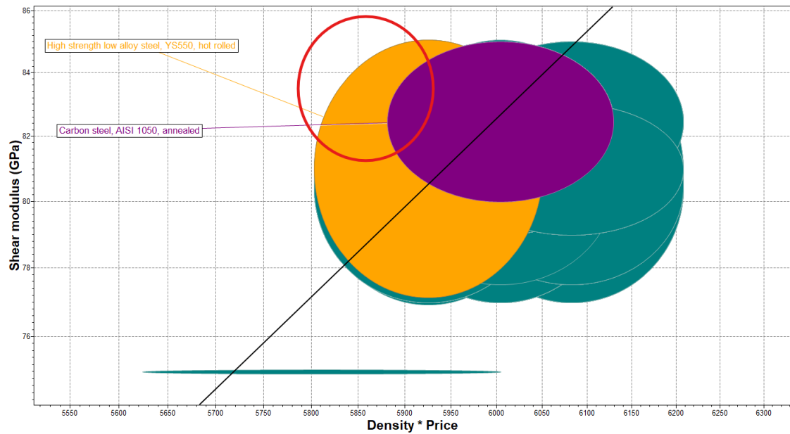
Figura 4: Diagrama de CES Edupack Para bulonería.
