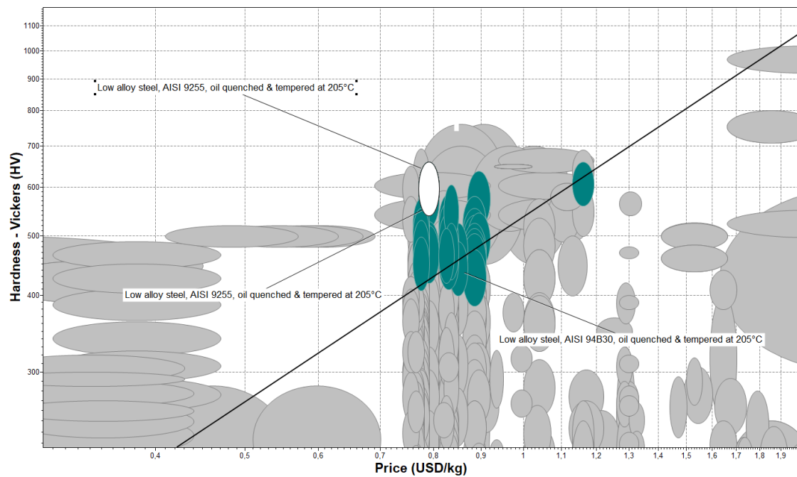
Figura 3: Diagrama de CES Edupack Para acero elegido para los cinceles.
