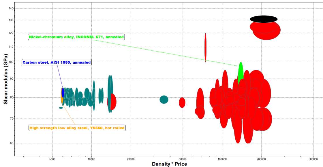
Figura 5: Diagrama N°2 de CES Edupack Para bulonería.
